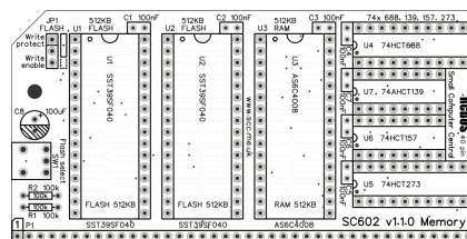
SC602 - Memory, 512kB + 2x512kB
