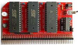
SC721 - Memory, 512kB + 2x512kB
