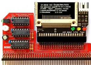
SC719 - Compact Flash
