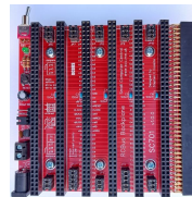
SC701 - Backplane, 6+1, 5 volt power
